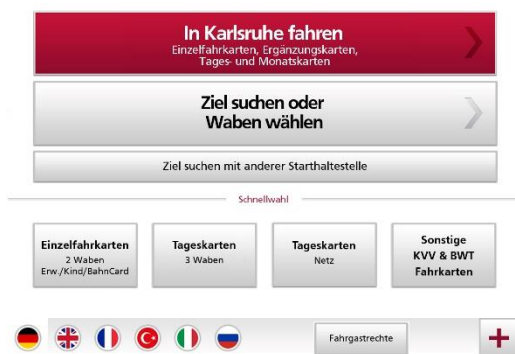
Abb. 1 aktuelle Startmaske
