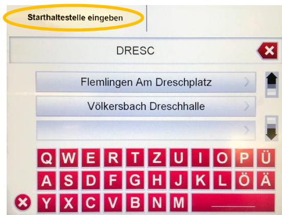
Abb. 4 Startwahlliste
